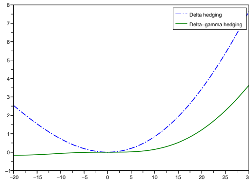
Figure 2.7: Sensibilité des positions couvertes en delta-gamma et en delta aux changements du prix de sous-jacent.
