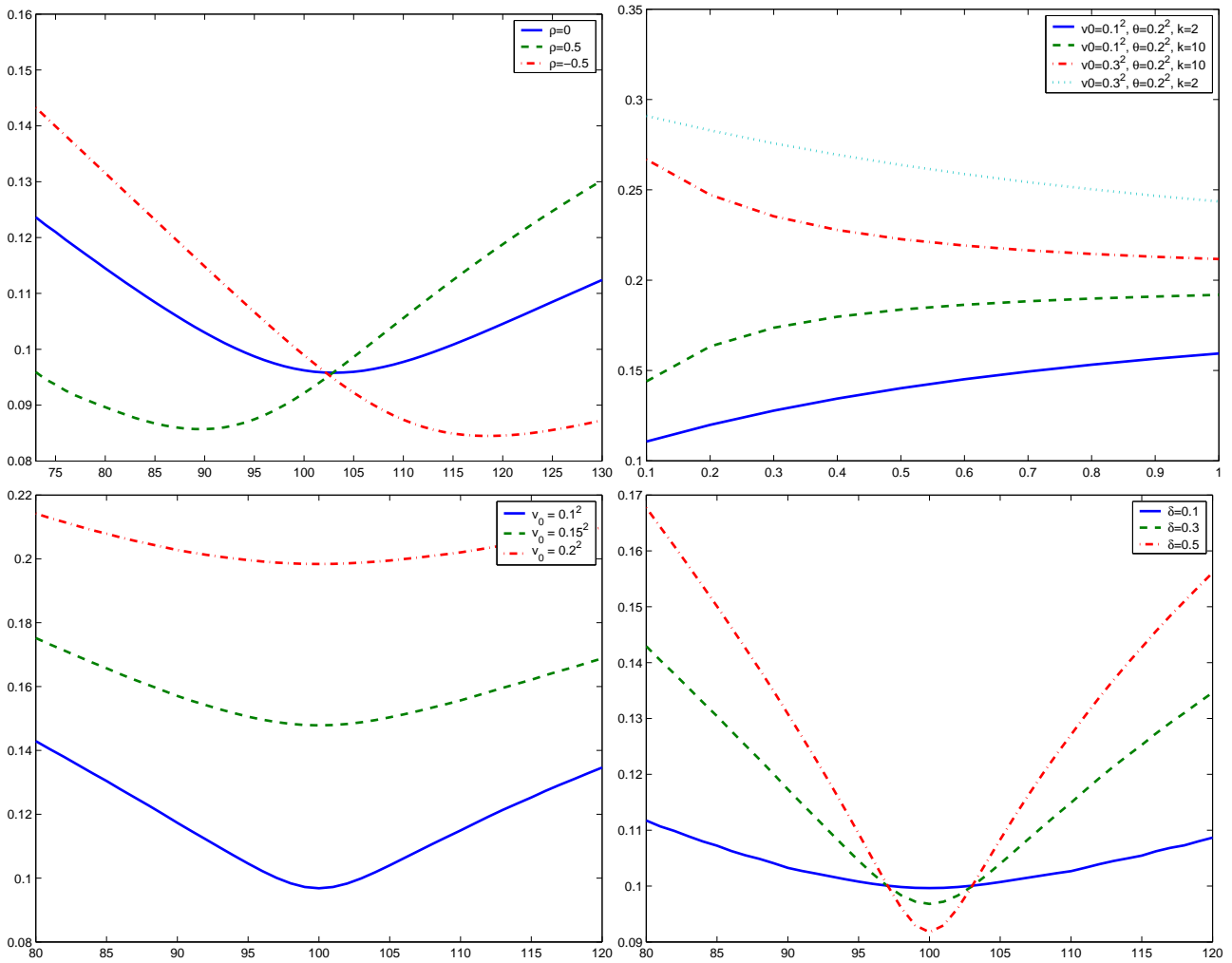
Figure 4.6: Influence de différents paramètres du modèle de Heston sur le comportement de la volatilité implicite. En haut à gauche: influence de la corrélation. En haut à droite: influence de k et \theta sur la structure par terme. En bas à gauche: influence du niveau initial de volatilité v_0 . En bas à droite: influence la volatilité de volatilité \delta .
