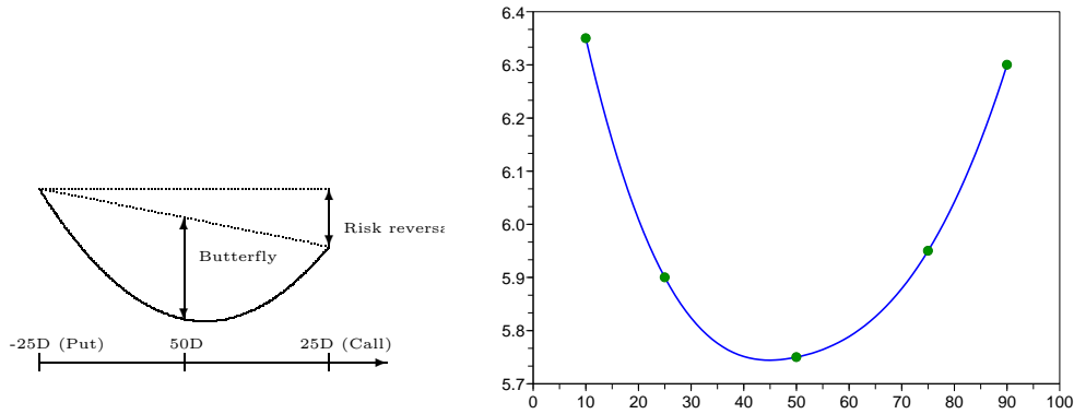
Figure 2.2: A gauche: représentation graphique des Butterfly et Risk Reversal. A droite: smile de volatilité pour les options sur EUR/USD de maturité 3 mois.
