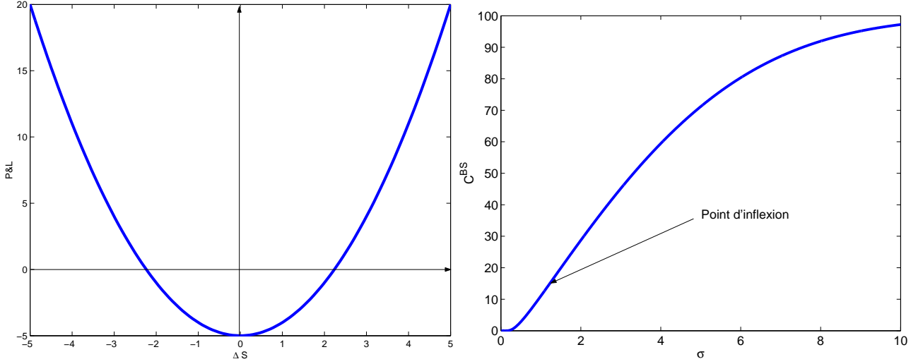
Figure 2.8: Gauche: la variation de la valeur d'une option couvert en delta après un changement du prix de sous-jacent de \Delta S . Droite: prix Black-Scholes d'une option en fonction de sa volatilité implicite.
