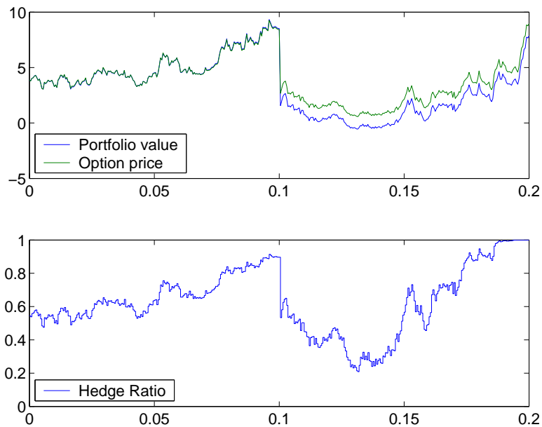
Figure 2.5: Effet d'un saut sur la stratégie de couverture. Rebalancement continu. P&L final = 1.10. Taille du saut : 7%.
