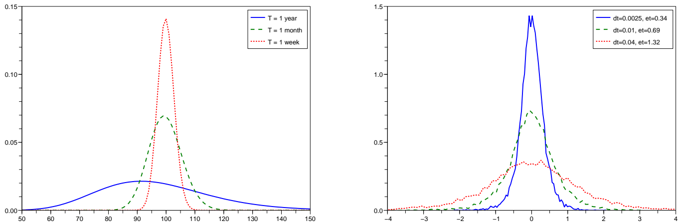
Figure 2.6: Gauche: gamma Black-Scholes d'une option call pour maturités différentes. Droite: histogrammes de l'erreur de couverture pour différentes fréquences de rébalancement.
